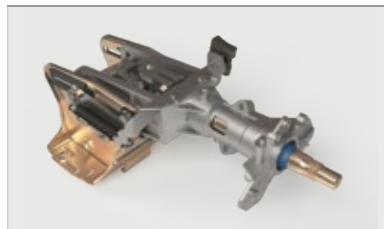
Рулевая колонка в сборе с распределителем 30104-3444000
