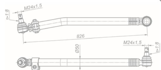
Тяга сошки с наконечниками 65201-3414010-60
