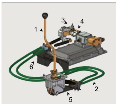
Привод управления КПП 536-1703003
