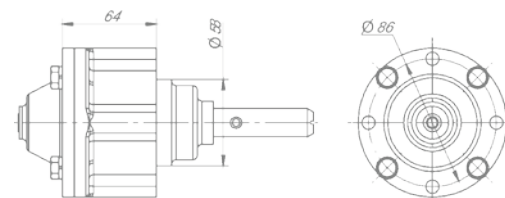
Механизм включения блокировки дифференциала РК 6522 19101-1803200
