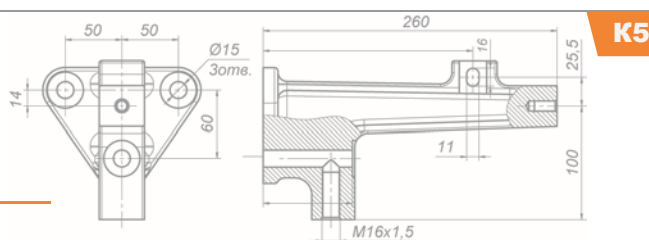
Кронштейн передней опоры кабины 65956-5001035-10
