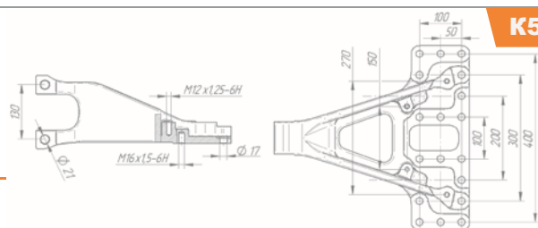
Кронштейн задней подвески 54901-2912447-10
