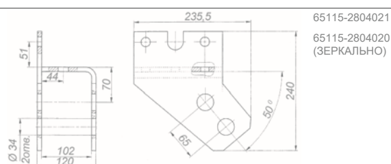
Кронштейн опорный 65115-2804020 (правый) 65115-2804021 (левый)
