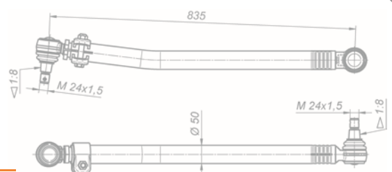
Тяга сошки с наконечниками 6520-3414010-41
