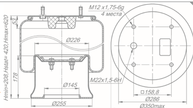
Рессора пневматической подвески 180-2934002-58
