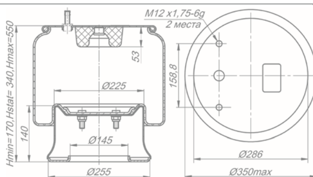
Рессора пневматической подвески 180-2934003-99
