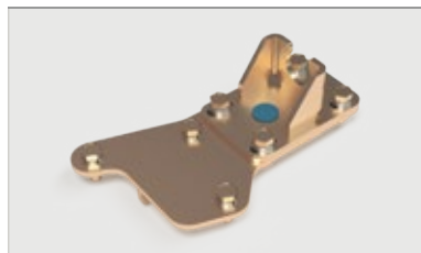
Кронштейн троса включения с крепежом 16108-1703320-10
