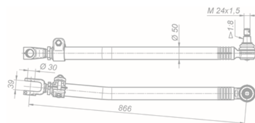
Тяга сошки с наконечниками 65225-3414010-11
