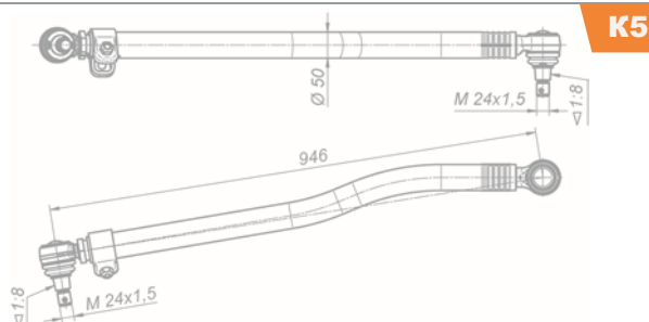
Тяга сошки 65952-3414010-20
