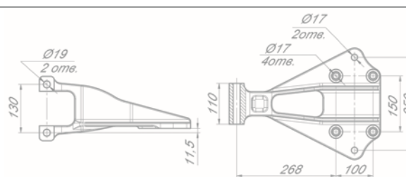
Кронштейн задней подвески R43083-2912445
