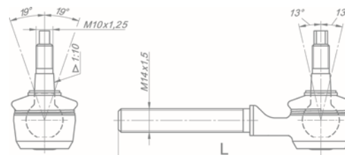
Хвостовик 362-1703420 (длинный L=120мм) 362-1703420-20 (короткий L=75мм)
