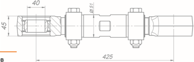
Штанга регулируемая 634-2919010
