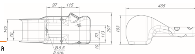
Кожух колонки передний 6520-3444073-19
