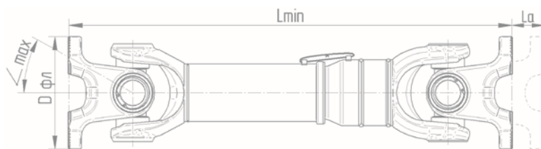
Карданные валы TD30
