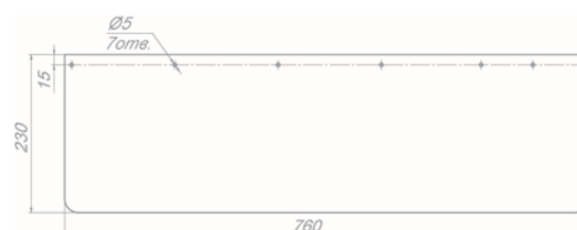
Брызговик облицовочной панели 43114-8401450-04
