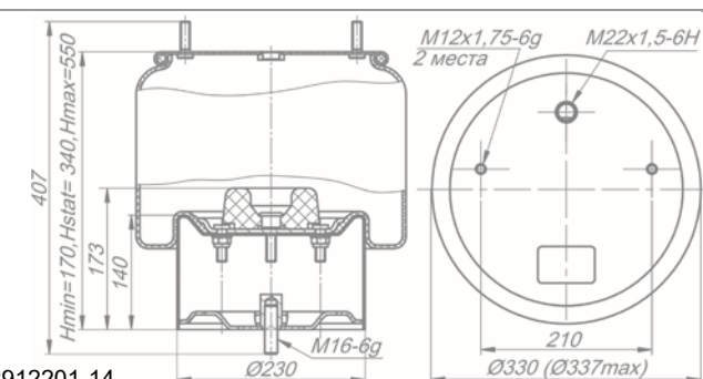
Рессора пневматической подвески 180-2934004
