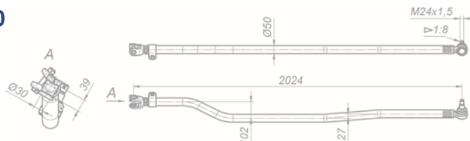
Тяга промежуточная 65808-3414130-20
