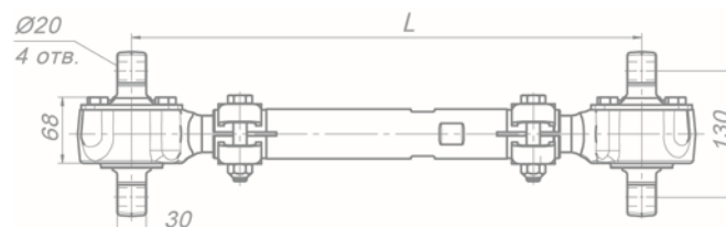
Штанга реактивная
