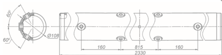
Буфер задний 65111-2804010
