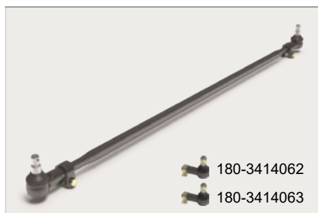
Тяга промежуточная 6540-3414130-11
