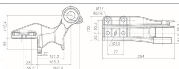
Кронштейн опорный правый R5490-5002042-10
