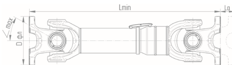
Карданные валы TD35
