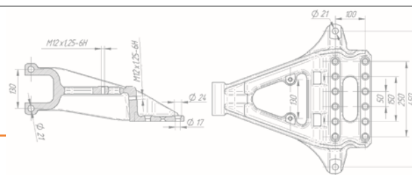
Кронштейн задней подвески 65206-2912445-47
