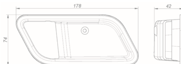
Накладка внутренней ручки замка двери левая 6520-6105189
