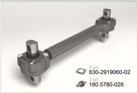
Штанга реактивная 632-2919010
