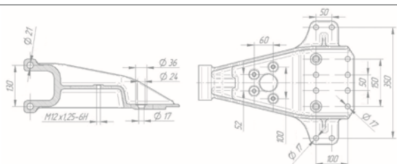
Кронштейн задней подвески 5490-2912445-45
