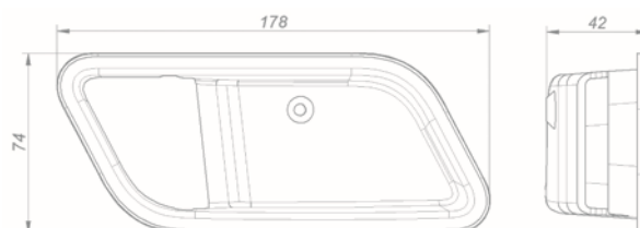
Накладка внутренней ручки замка двери правая 6520-6105188
