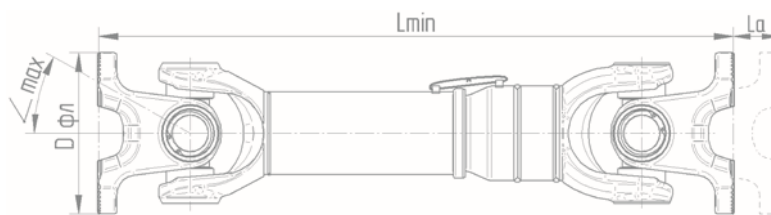
Карданные валы TD14
