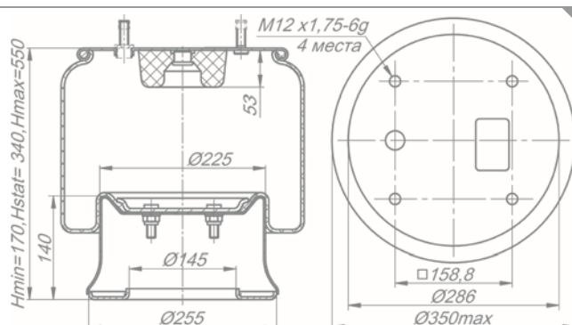
Рессора пневматической подвески 180-2934002-99
