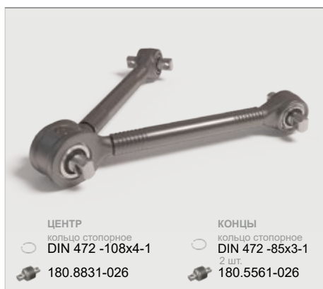
Штанга V-образная 1515-2919012-40
