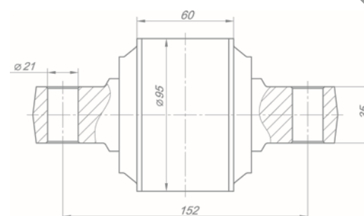
Резинометаллический шарнир 6520-2919026
