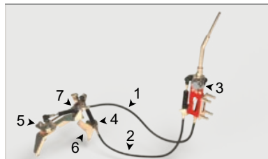
Тросовый привод переключения КПП 16506-1703000-10
