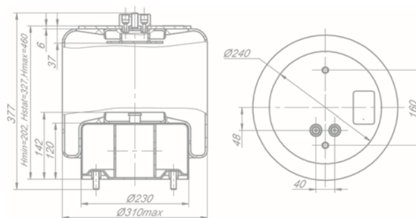
Рессора пневматической подвески 651-2934002-56
