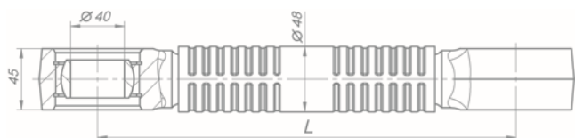
Штанга реактивная
