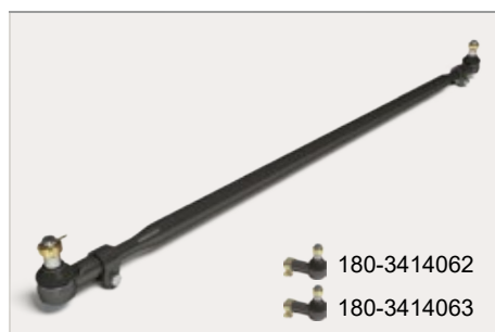
Тяга промежуточная 65228-3414129-11
