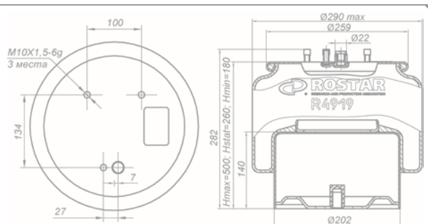
Рессора пневматической подвески 180-2934002-105
