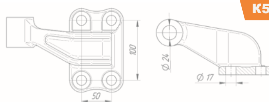
Кронштейн амортизатора верхний 65951-2905510 (правый) 65951-2905511 (левый)
