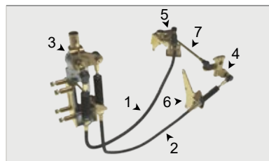
Тросовый привод переключения КПП 16506-1703000
