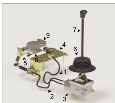
Привод управления КПП 16105-1703000
