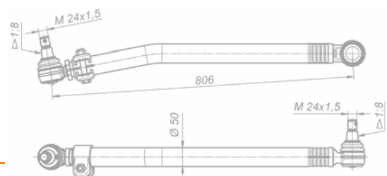
Тяга сошки с наконечниками 6460-3414010-60
