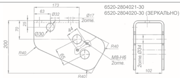
Кронштейн опорный 6520-2804020-30 (правый) 6520-2804021-30 (левый)
