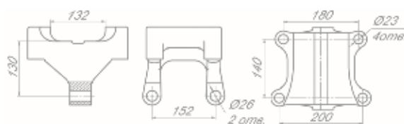
Рычаг нижний задний правый R65117-2919182
