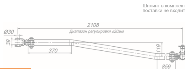
Тяга промежуточная 65201-3414129-51
