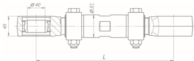
Штанга реактивная 634-2919010-11 634-2919010-23 634-2919010-24 634-2919010-25 634-2919010-26
