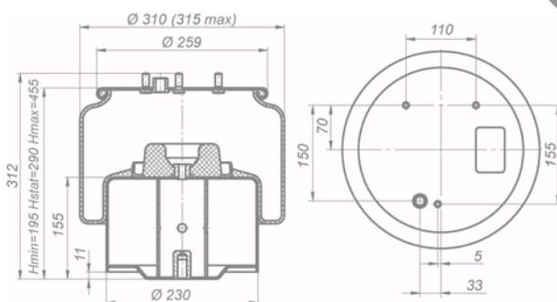
Рессора пневматической подвески 180-2934002-35
