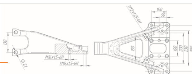
Кронштейн задней подвески 5490-2912447
