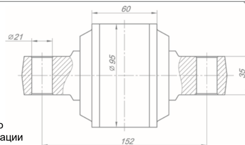
Резинометаллический шарнир 5460-2919026-40
