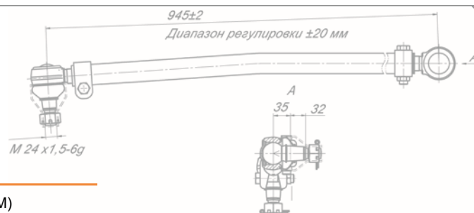
Тяга продольная 180-3414010-141
