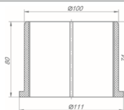
Комплект втулки башмака балансира 55111-2918074-01K
