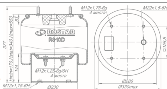
Рессора пневматической подвески 180-2934004-99
