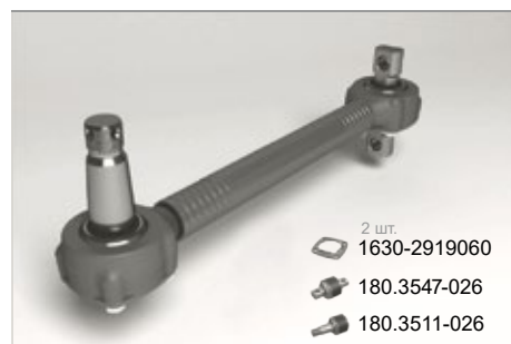
Штанга реактивная 1630-2919010-10 1630-2919010-11 1630-2919010-12
