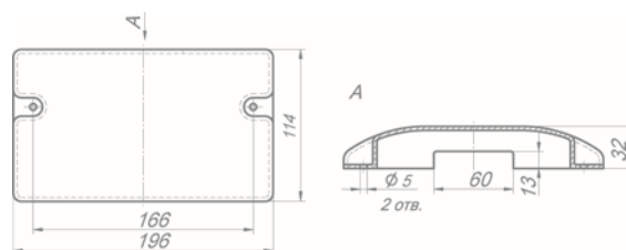
Крышка инерционной катушки 53205-5401071
