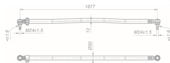
Тяга рулевой трапеции 4308-3414052
