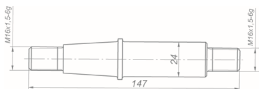
Палец крепления амортизатора P53212-2905418
