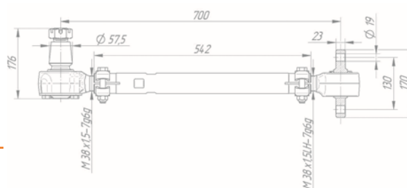
Штанга задней подвески верхняя 529265-2919014-03
