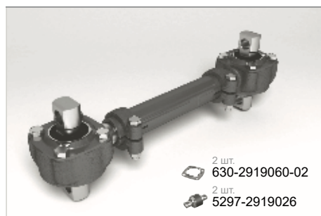
Штанга реактивная
