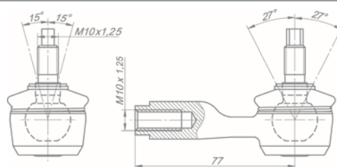
Наконечник 362-1703521-20 (правый) 362-1703522-20 (левый)
