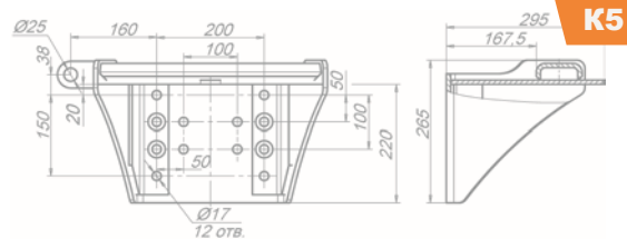
Кронштейн пневморессоры подвески верхний R65659-3011050 (правый) R65659-3011051 (левый)
