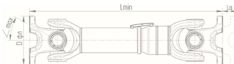
Карданные валы TS25
