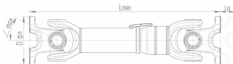
Карданные валы TD25
