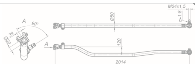
Тяга промежуточная 65801-3414130-20
