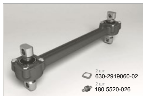
Штанга реактивная 1631-2919012 1631-2919012-10 1631-2919012-20
