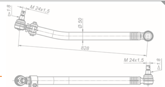
Тяга сошки с наконечниками 6520-3414010-51
