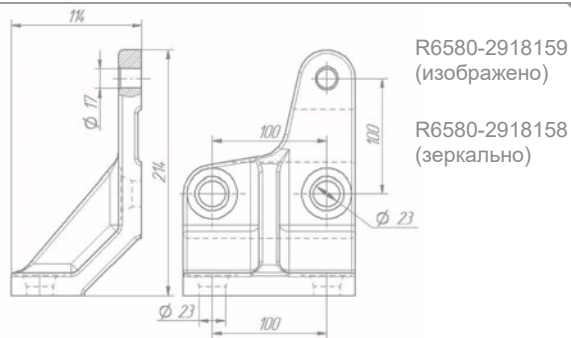
Вставка лонжерона R6580-2918158 (правая) R6580-2918159 (левая)
