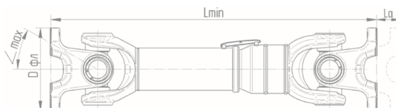
Карданные валы TD17
