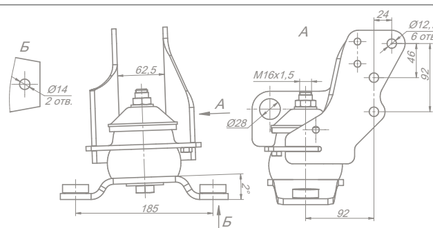
Опора передняя правая 650.1001019-30
