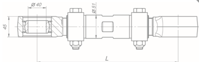
Штанга реактивная 634-2919010-10 634-2919010-20 634-2919010-21 634-2919010-22
