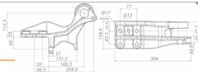
Кронштейн опорный левый R5490-5002043-10
