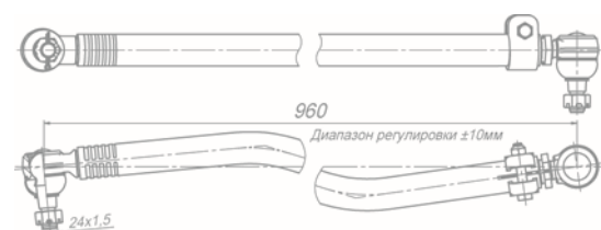
Тяга рулевая продольная 180-3414010-220
