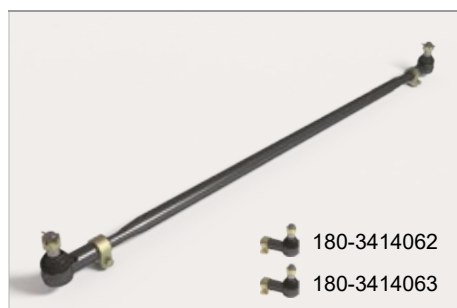
Тяга промежуточная 6350-3414129-11
