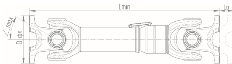
Карданные валы TS35
