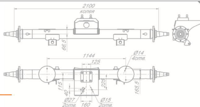
Балка оси R65208-3011500-03
