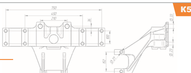
Кронштейн оси балансира 65956-2918056
