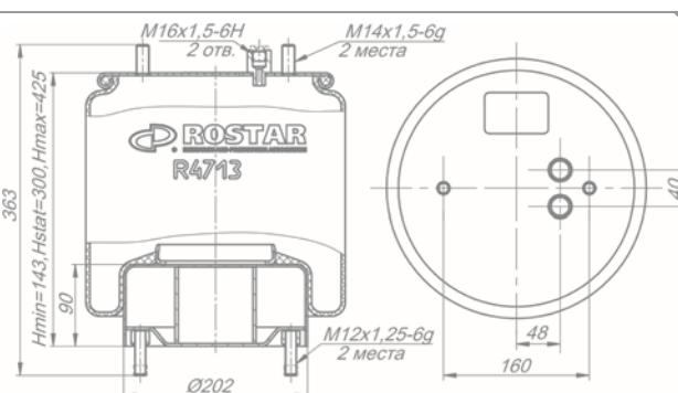
Рессора пневматической подвески 180-2934003-23
