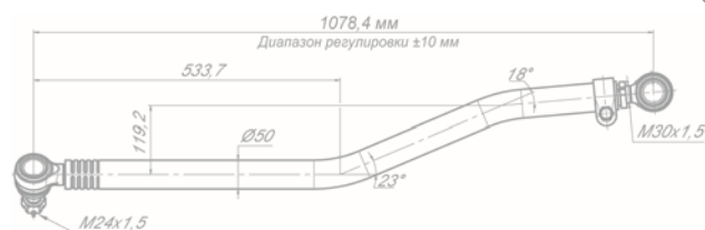
Тяга рулевая продольная 180-3414010-481
