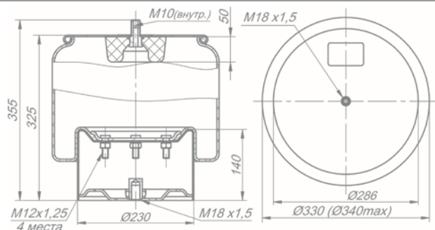
Рессора пневматической подвески 180-2934002-03
