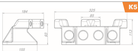
Кронштейн реактивной штанги верхней задний R65659-3011190
