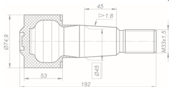
Шарнир реактивной штанги 210-2919026
