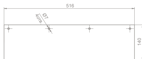
Фартук щитка грязевого верхнего 65226-8403295-10
