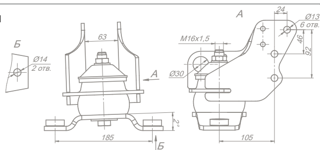
Опора передняя правая 650.1001019-20
