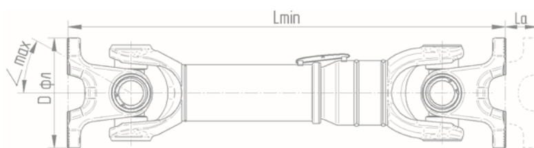
Карданные валы TS30
