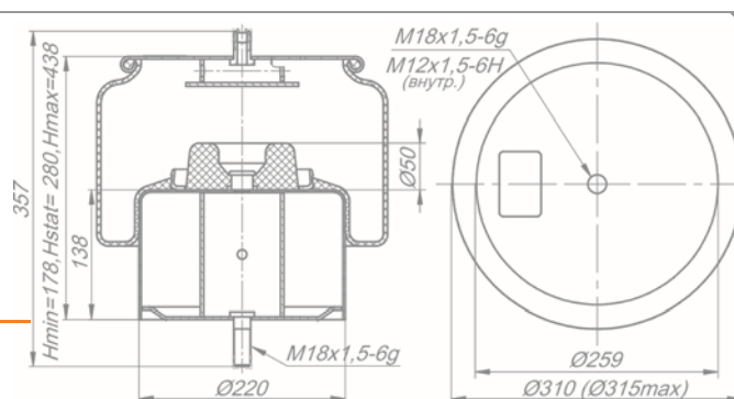
Рессора пневматической подвески 180-2934003-33
