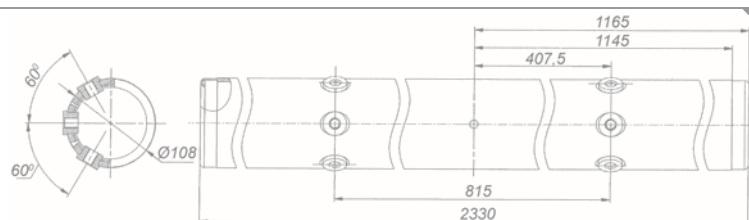
Буфер задний 65115-2804010
