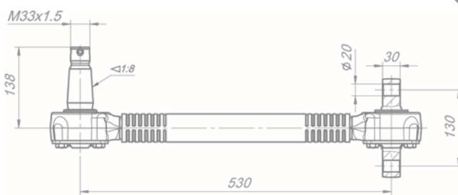
Штанга реактивная 1630-2919010-10 1630-2919010-11 1630-2919010-12
