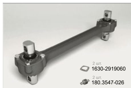
Штанга реактивная 1630-2919012
