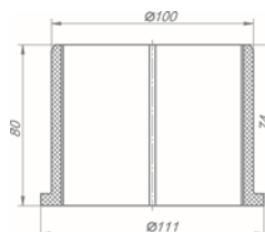
Комплект втулки башмака балансира 55111-2918074-013
