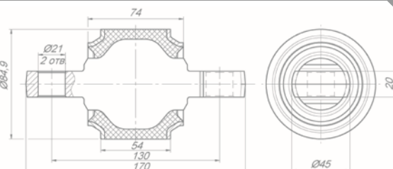
Шарнир реактивной штанги
