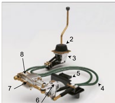
Комплект тросового привода переключения КПП 530-1703000
