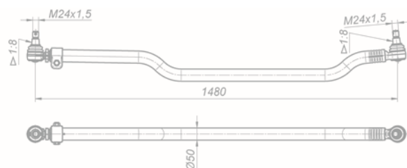
Тяга рулевой трапеции 5350-3414052
